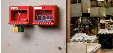
S3650 comes with 1 lock box and 1 mounting bracket Safety padlocks sold separately. S3650 umfasst 1 Verriegelungskasten und 1 Halterung Sicherheitsvorhängeschlösser separat erhältlich
